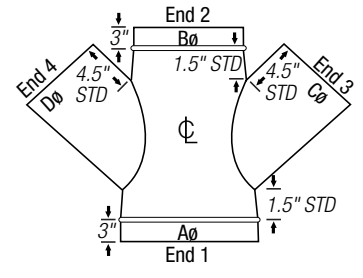
(D) Double Wye Branch with Collars
