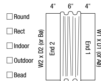
(D) Flex Connector
